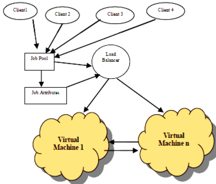
Fig. 2 ESCE Algorithm
