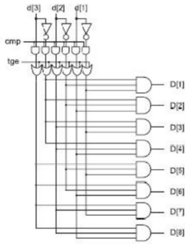
Fig.3. 3x8 decoder
