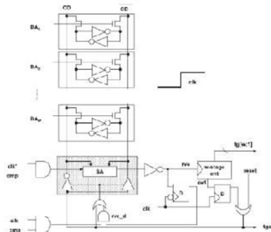
Fig.4. Logic module
